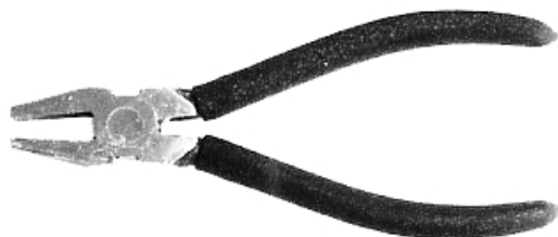
32 132 00 PROVETRO - lámací klešty PCJ-3, délka 165 mm, šířka čelistí 10 mm, určeno pro sílu skla 2 - 6 mm
