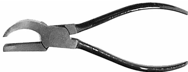
32 118 20 PROVETRO P410 - speciální lámací kleštky určené především pro lámání zrcadloviny, délka 185 mm, šířka čelistí 15 mm, ideální pro sílu skla 3 - 16 mm
