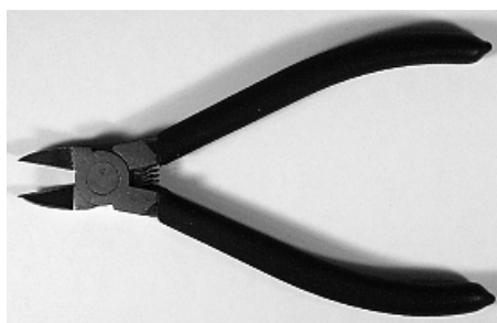
32 170 00 PROVETRO PLP 7 - kleštky na štípání olověných profilů
