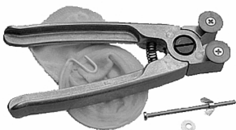
32 160 00 ZAG-ZAG - klešťa mosaikové, typ 701.0 32 160 01 Kolečko lámací - náhradní 32 160 02 Sítaek plátěný na sklo - náhradní
