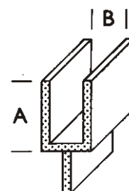
Profil U krajový s praporkem ve středu profilu pro vsazování vitráží do dvojskel
