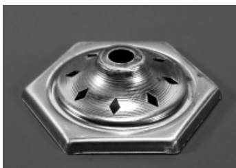
22 282 00 kapna mosaz, šestiúhelník s otvory, délka hrany : 42 mm
