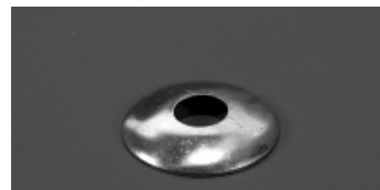
22 100 00 kapna mosaz průměr : 3,0 cm, průměr otvoru : 5 mm
