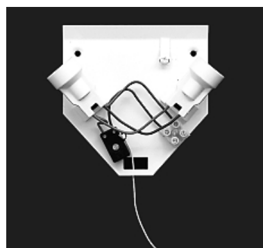
20 261 02 montura nástěnná E 14, dvojobjímková s vypínačem
