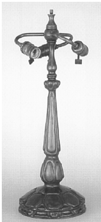
89 LB 587 MOCKTURTLE BASE h: 55 cm / 22" für Schirmdurchmesser: 40 - 46 cm fits shades 16" - 18"
