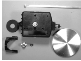
55 110 00 Quarzuhrwerk mit Pendel Quartz clockwork with pendulum
