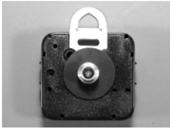
55 100 00 Quarzuhrwerk / Quartz clockwork Länge Uhrenwelle Shaft = 12,5 mm
